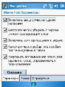
Экран Options/Параметры
