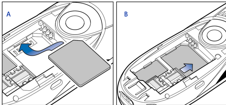
Рис. 1 Расположение и фиксация карты памяти
