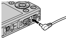
Фиксатор аккумулятора Переходник постоянного тока DR-10
