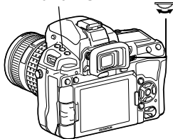
Увеличение выдержки
