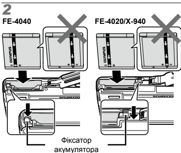
Кришка акумуляторного відсіку/картки
