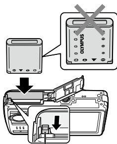
Фіксатор акумулятора
