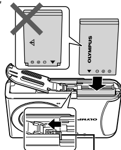
Ручка фиксатора аккумулятора
