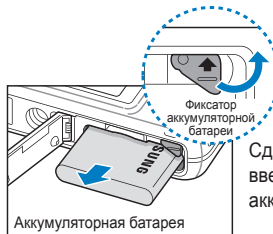
Аккумуляторная батарея
