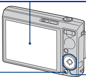
Кнопка HOME
