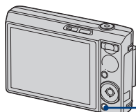
Кнопка HOME
