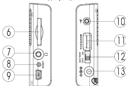
Вид справа/слева
