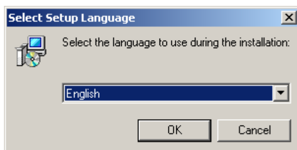
Рис. 9: Выберите язык
