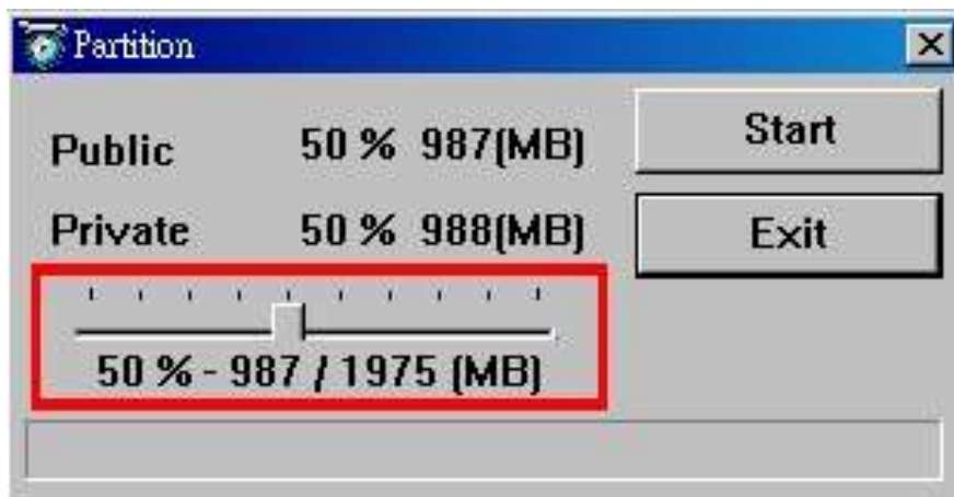
Рис. 18: Сегментация памяти
