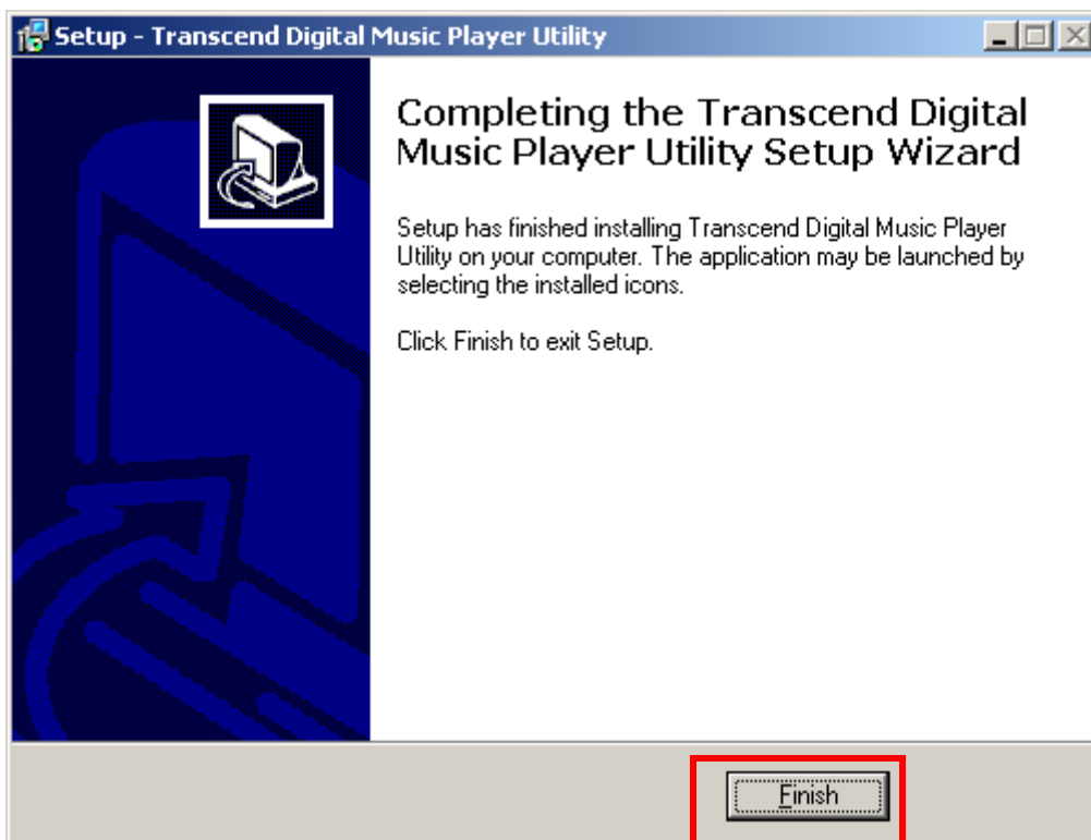
Рис. 11. Установка закончена
